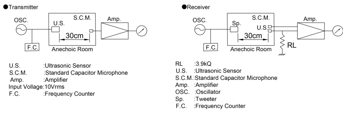
图 1: 典型测试电路
