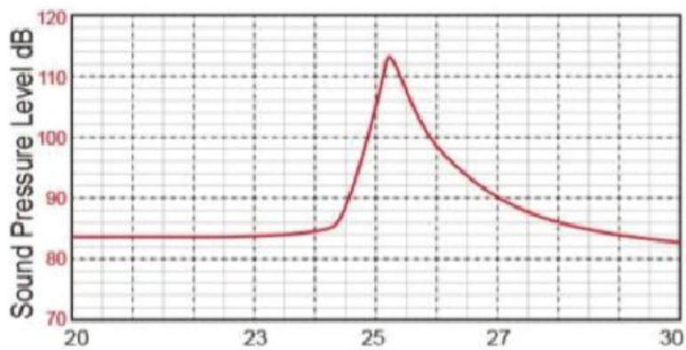
图 3: 声压灵敏度
