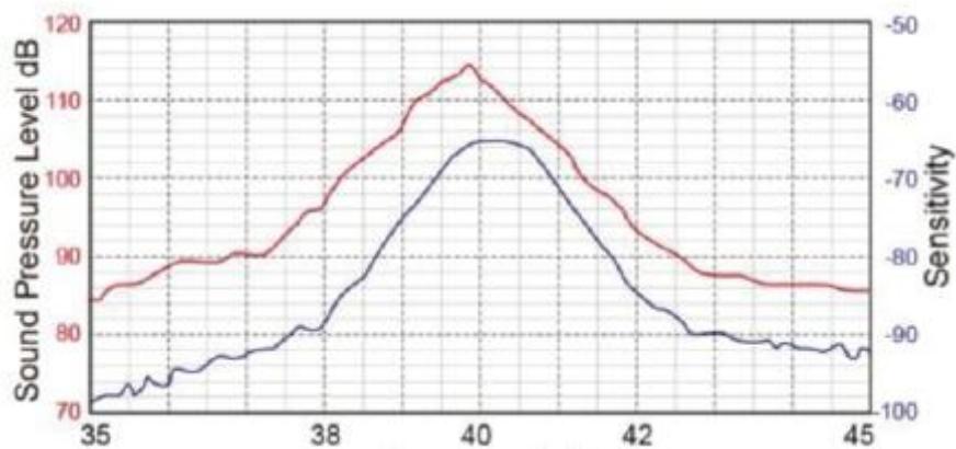
图 3: 声压灵敏度
