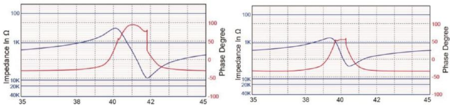
图 2: 阻抗幅度/相位
